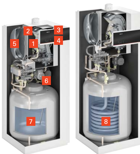
VITODENS 111-F (typ B1TF)
